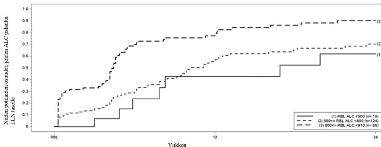
Kuva 1: Kaplan–Meierin menetelmällä arvioidut niiden potilaiden osuudet, joiden absoluuttinen lymfositimäärä (ALC) palautui palautumisen lähtötilanteesta (RBL) normaaliarvojen alarajaan (LLN) ( \geq 910 solua/mm 3 )
