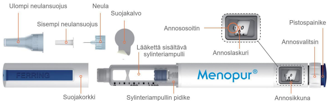
Menopur esitäytetty kynä ja sen osat
